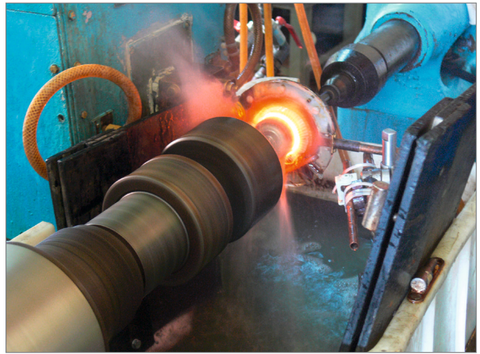
Induktionshärten in der Härterei TANDLER
